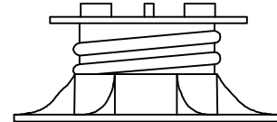
SE4 2" - 3"
